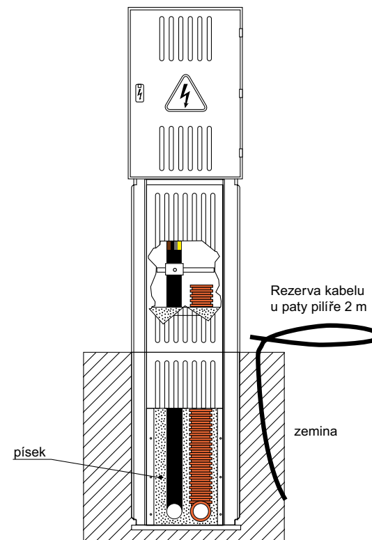
Obr. 2 Přípojková skříň v pilíři se založenou chráničkou
