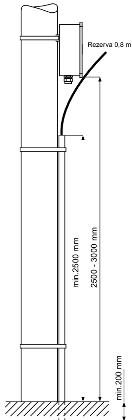
Obr. 1 Přípojková skříň na podpěrném bodu
