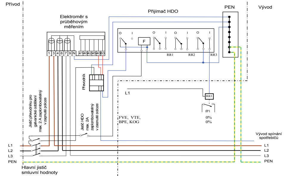
13. Schéma zapojení měření s přímým třífázovým elektroměrem s převodníkem, regulací činného výkonu OZE a přijímačem HDO (od Prez 0 kW do 100 kW včetně)
