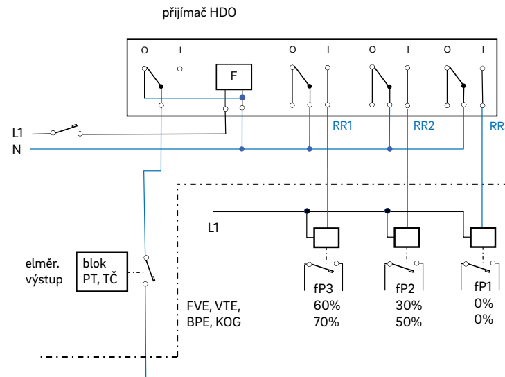
14. Zapojení přijímače HDO pro regulaci výkonu OZE
