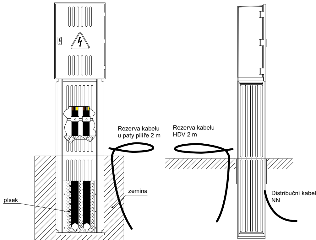
Obr. 3 Stávající přípojková skříň bez založené chráničky
